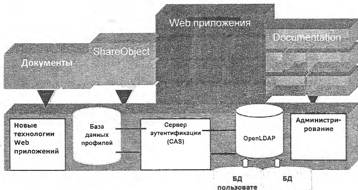
Рис. 1. Архитектура идентификационной системы на открытых кодах.
